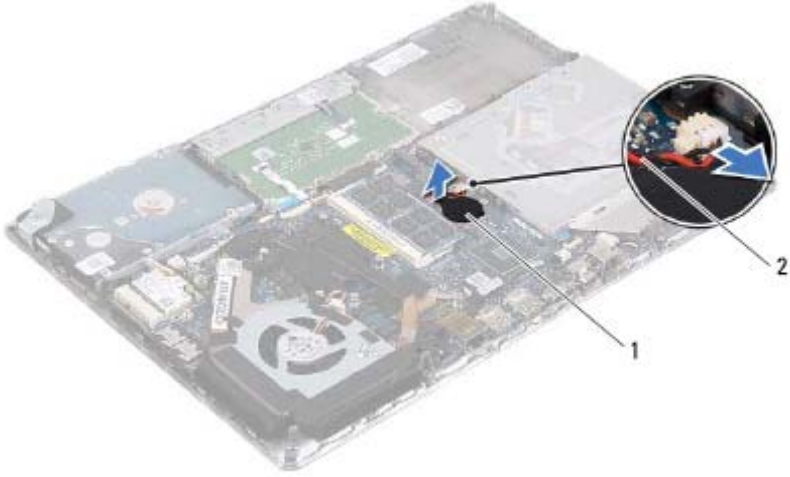
1 البطارية الخلوية المصغرة 2 كبل البطارية الخلوية المصغرة
